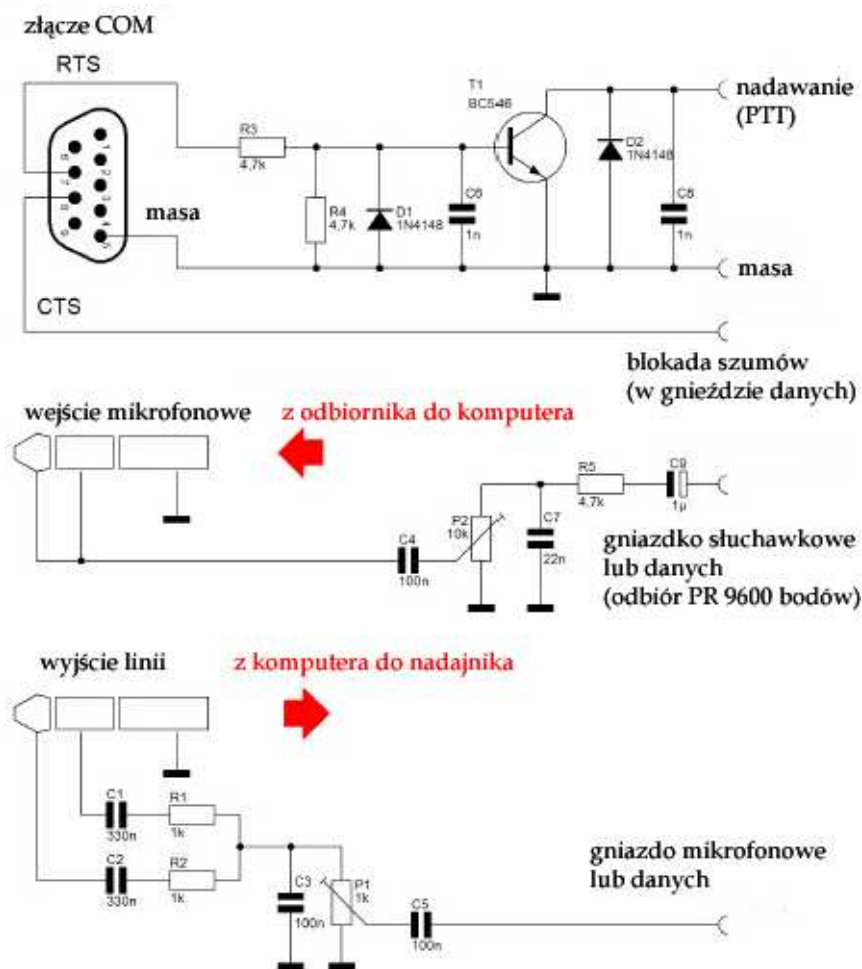
Rys. 2.2. Inny wariant prostego układu pośredniczącego. Do kluczenia nadajnika zamiast optoizolatora zastosowano tranzystor wykonawczy npn. Wzorując się na układzie poprzednim można i tutaj dodać optyczną sygnalizację nadawania na diodzie świecącej i wykorzystać do kluczenia również przewód DTR.
